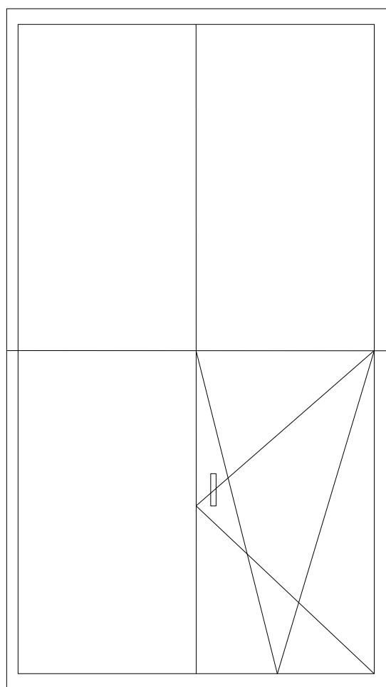
Окно: 2030мм x 660мм (h) - 3 шт.
